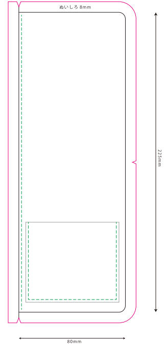
【型紙⑤サイドポケット/右】
