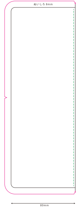
【型紙③サイドポケット/左】
