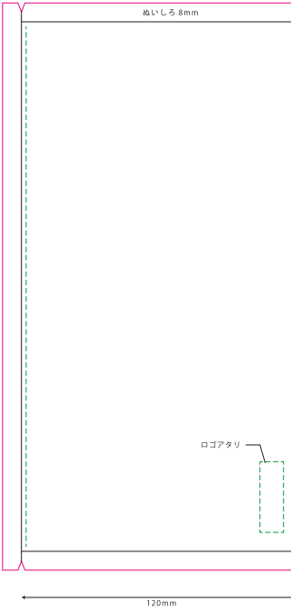
【型紙④底面】
