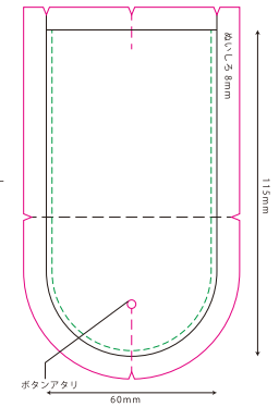
【型紙⑧フラップ】×2枚
